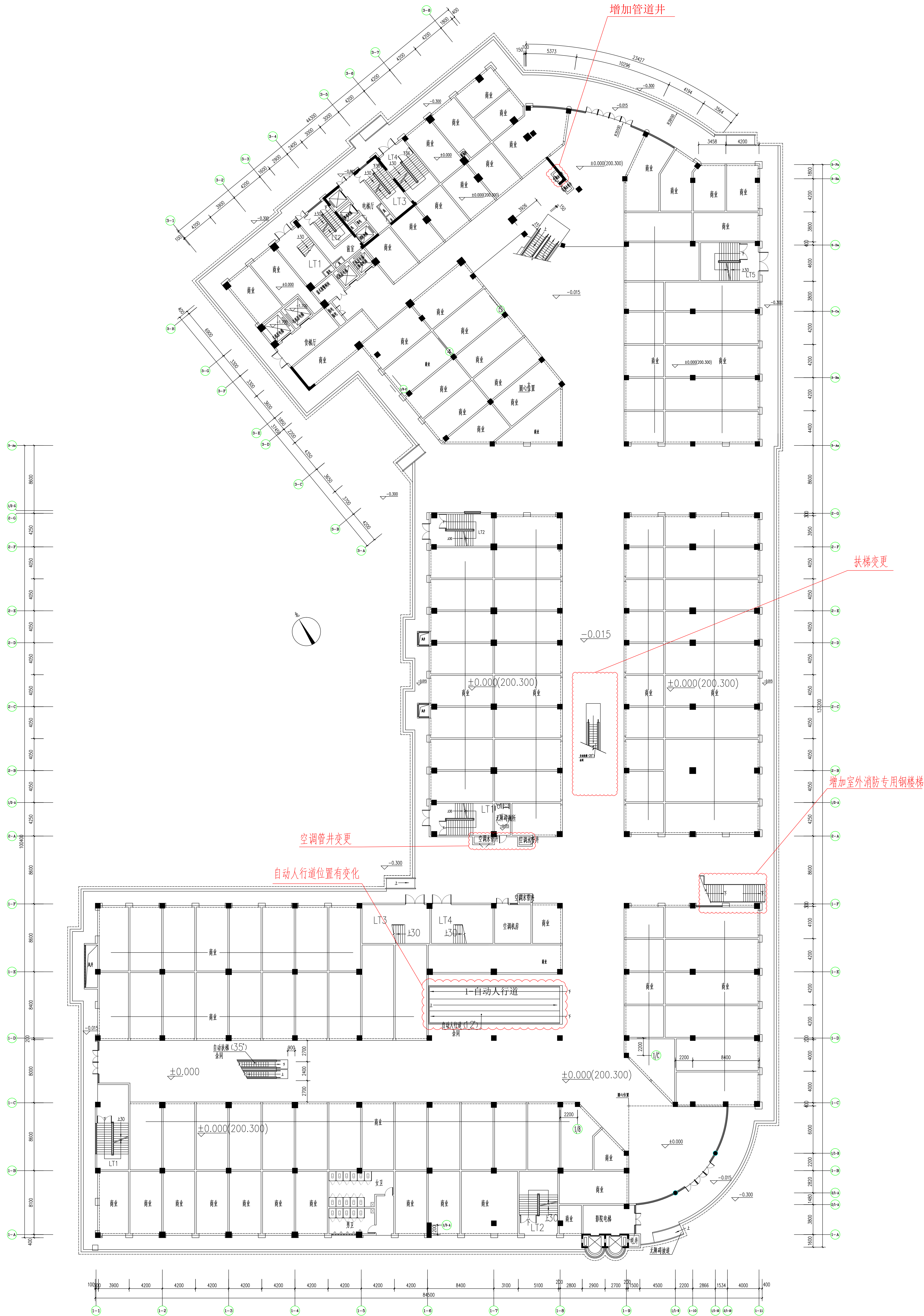
一层平面图
